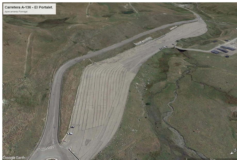
Vista disponible en Google Earth del aparcamiento de la estación de esquí de Formigal, próximo a El Portalet en la carretera A-136, donde es fácil apreciar la magnitud de los movimientos en masa de carácter lento.
